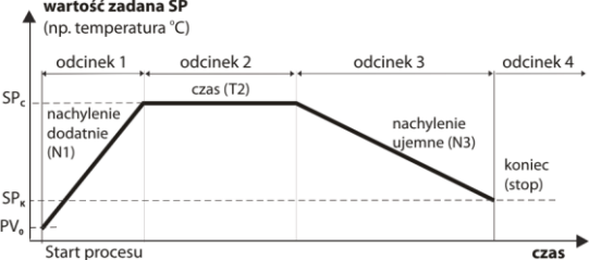
Rys.12.4.3.1. Schemat przykładowego programu.
