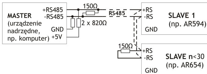
Rys.17. Schemat poglądowy sieci RS485
