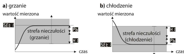
Rys.13.5. Położenie strefy nieczułości dla grzania (8: AutE = Auto ) oraz chłodzenia (8: AutE = Chl )
